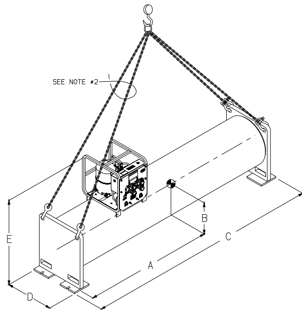
Fig. 4 — Rigging Guide
