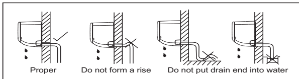
Fig. 18 — Installation appropriée du flexible d'évacuation
