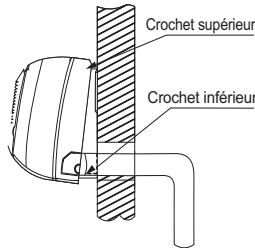
Fig. 13 – Installation du module intérieur
