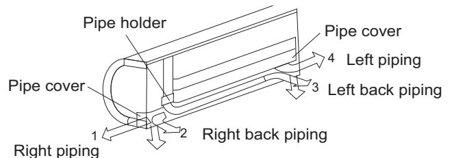
Fig. 9 – Emplacements des tuyauteries
