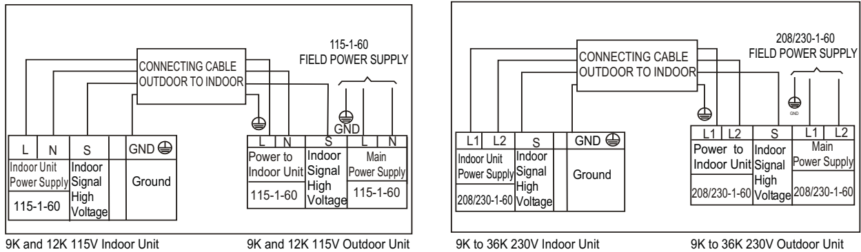
Fig. 10 – Schémas de raccordement
