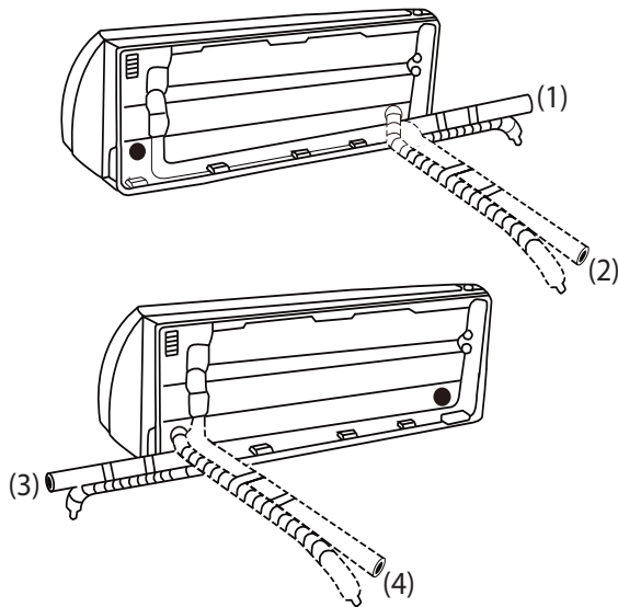
Fig. 8 – Emplacement de sortie de la tuyauterie
