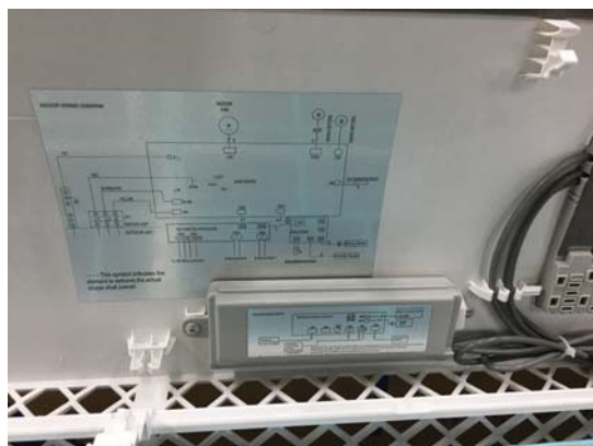
Fig. 27 – Installation de la carte multifonction
