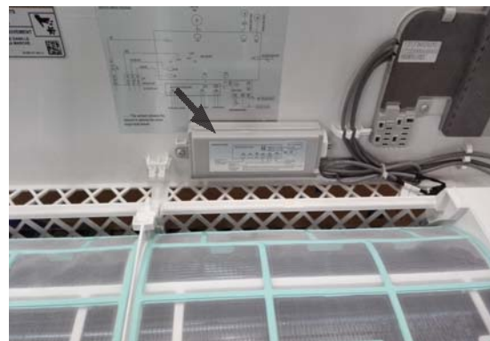
Fig. 22 — Carte multifonction
