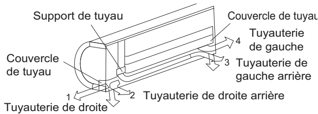
Fig. 7 – Emplacements des tuyauteries
