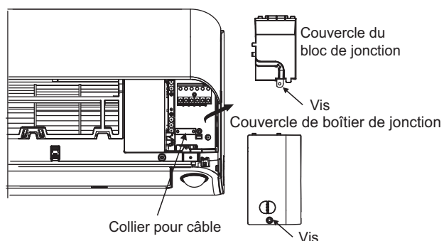
Fig. 13 – Emplacement du bloc à bornes
