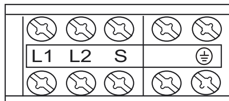
Fig. 14 – Câblage d'alimentation et de commande du module intérieur
