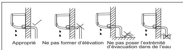
Fig. 20 — Installation appropriée du flexible d'évacuation
