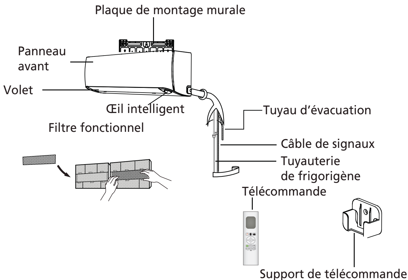
Fig. 1 – Liste de pièces
