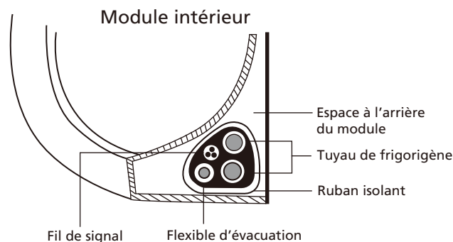
Fig. 21 — Regroupement du flexible d'évacuation, de la tuyauterie de frigorigène et du câble de signal
