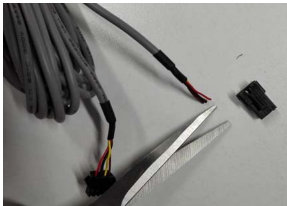
Fig. 25 – Coupe de la prise femelle et dénudage des fils
