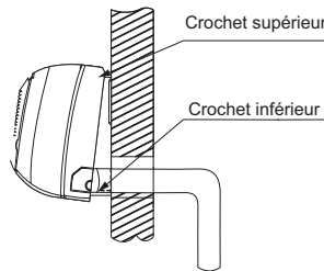
Fig. 15 – Installation du module intérieur
