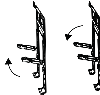
Fig. 10 – Utilisation du support pour le soutien du module
