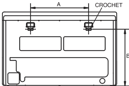
Figure 10 — Emplacements des crochets de montage
