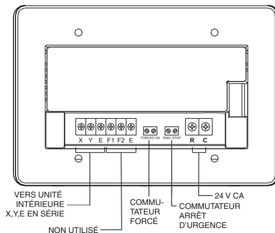
Figure 16 — Câblage du contrôleur central
