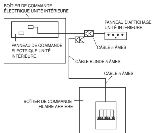
Figure 15 — Câblage de la télécommande filaire (non programmable)
