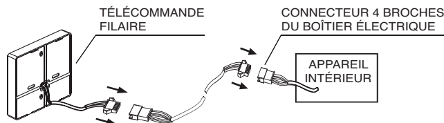
Figure 14 — Câblage de la télécommande filaire (programmable)
