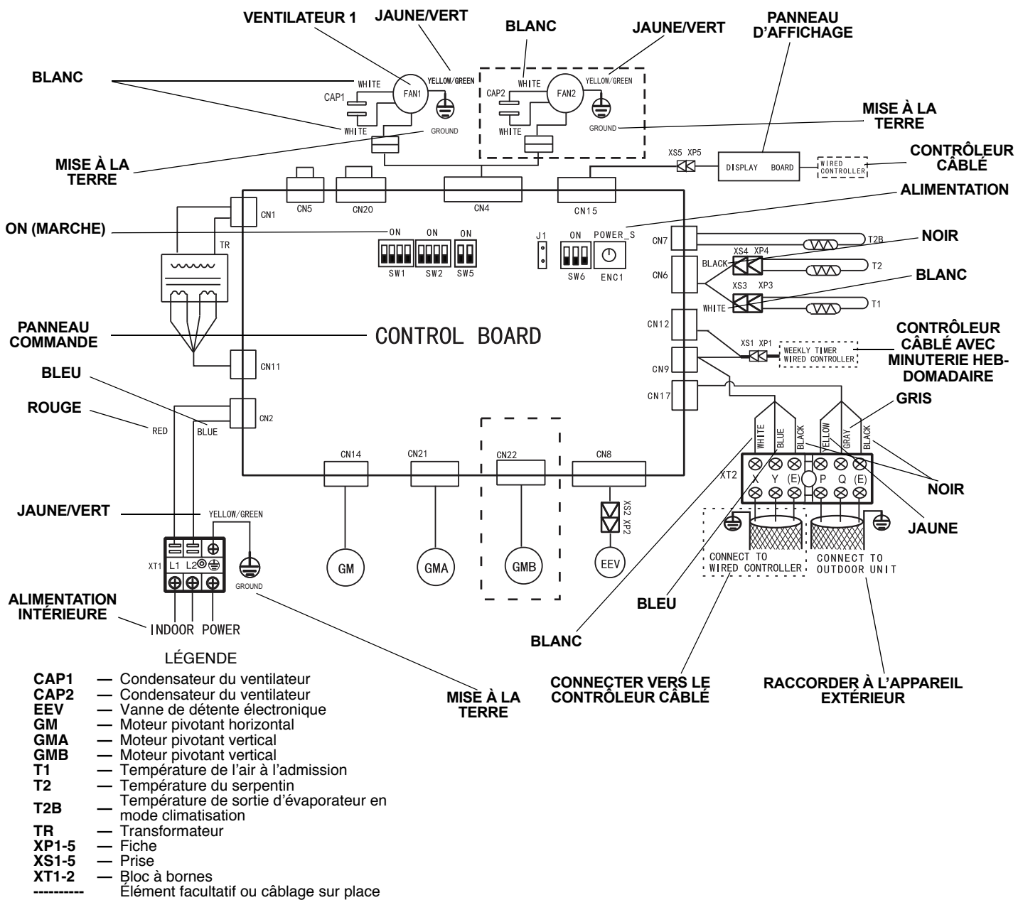
Figure 12 — Schéma du câblage type des appareils 40WAU012-048
