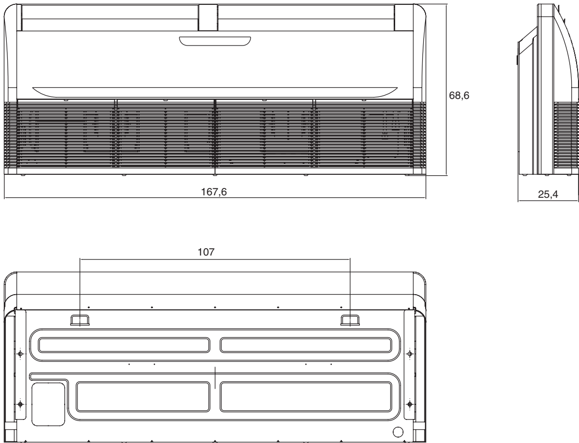
Figure 3 — Dimensions des appareils 40WAU 036 et 048
