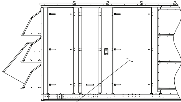
ERV SECTION ACCESS DOOR
