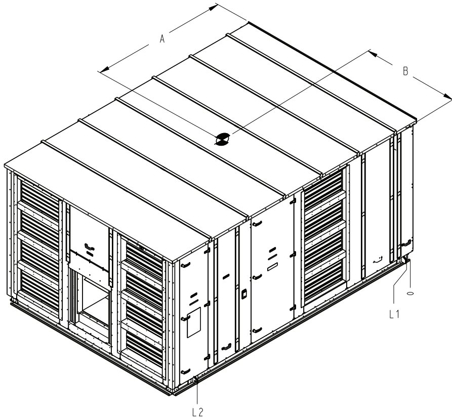
Fig. 28 — 48N 75-150 Ton Split (ERV Section) Rigging
