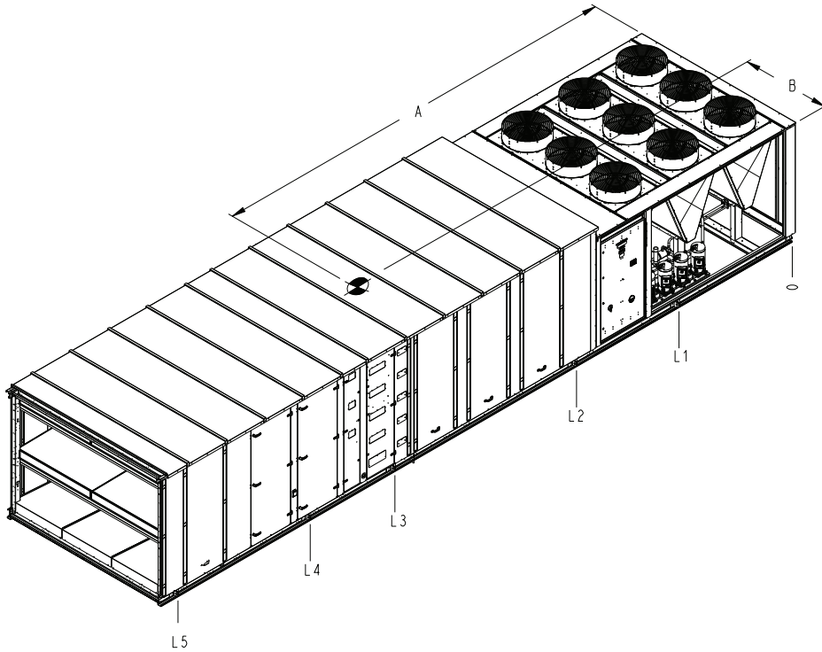
Fig. 26 — 50N 75-150 Ton Split (Main Unit) Rigging
