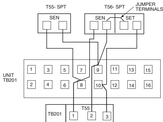
Fig. 71 — T-55 or T-56 Wiring
