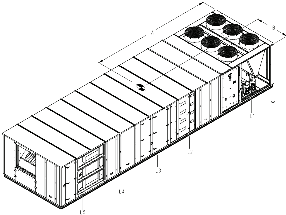
Fig. 25 — 50N 75-150 Ton Non-Split Rigging
