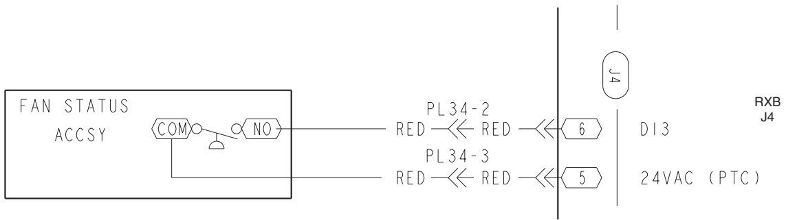
Fig. 77 — Fan Status Switch Wiring
