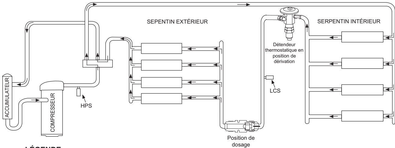
Figure 12 – Carte de dégivrage
