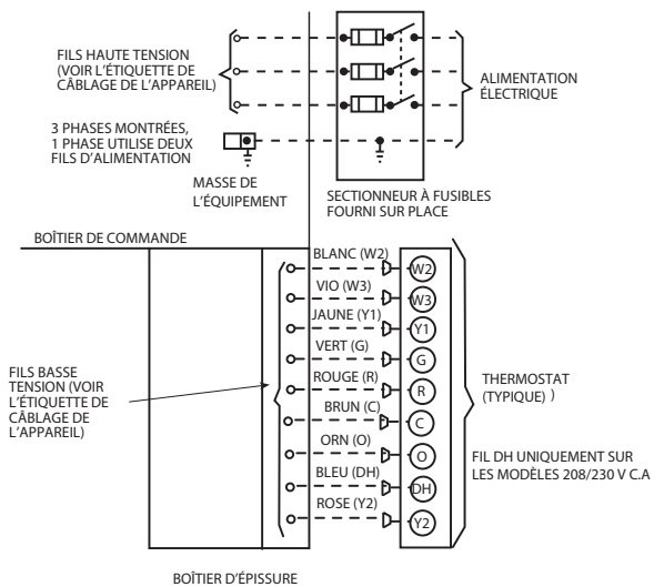
Figure 10 – Branchements haute et basse tensions
