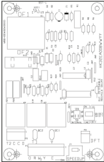
Figure 12 – Carte de dégivrage
