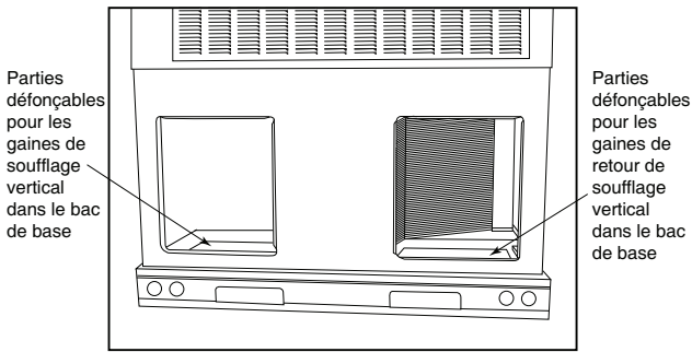
Figure 9 – Ouvertures d’air de soufflage et de retour
