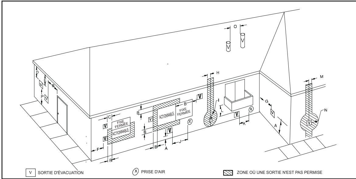
Figure 52 – Dégagement des sorties d'évent d'un système à ventilation directe
