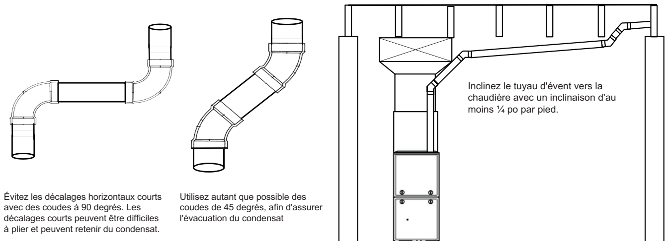
Figure 43 – Raccordement des événements près de la chaudière
