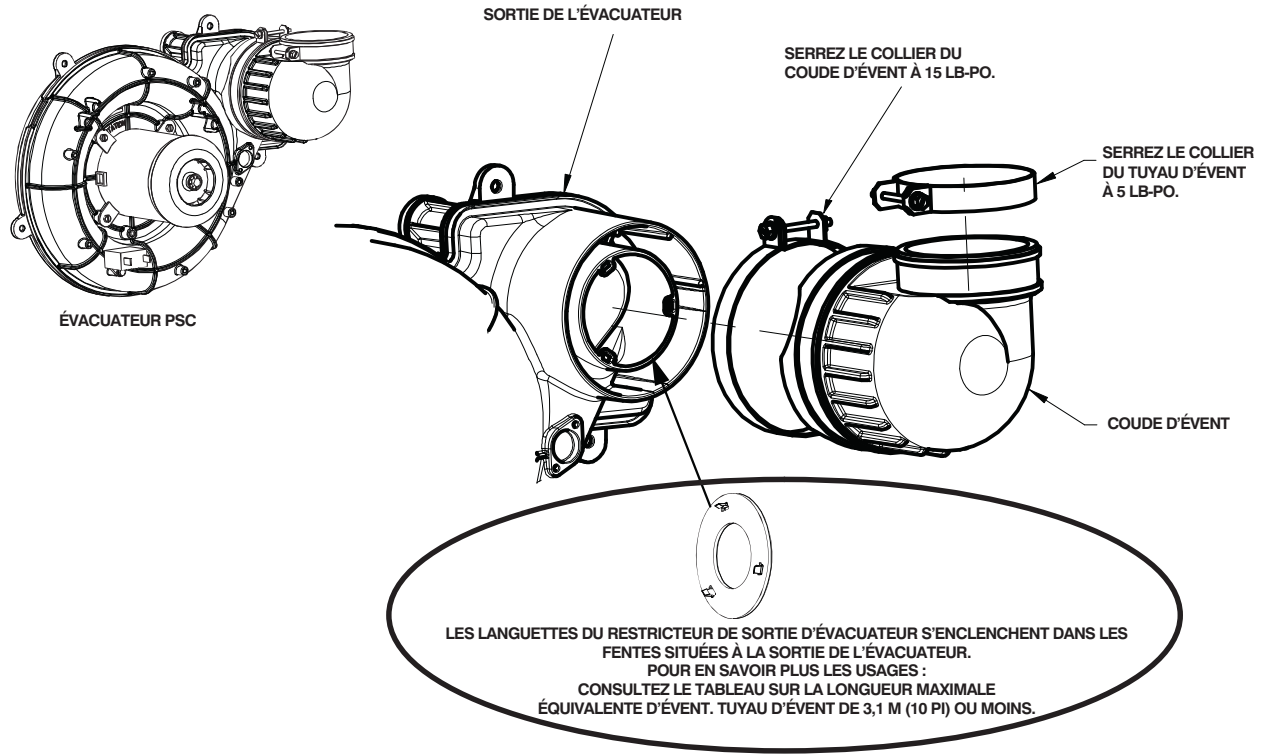
Figure 42 – Coude d'évent d'évacuateur
