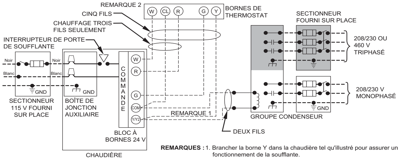
Figure 39 – Schéma de câblage type d'un appareil à une phase
