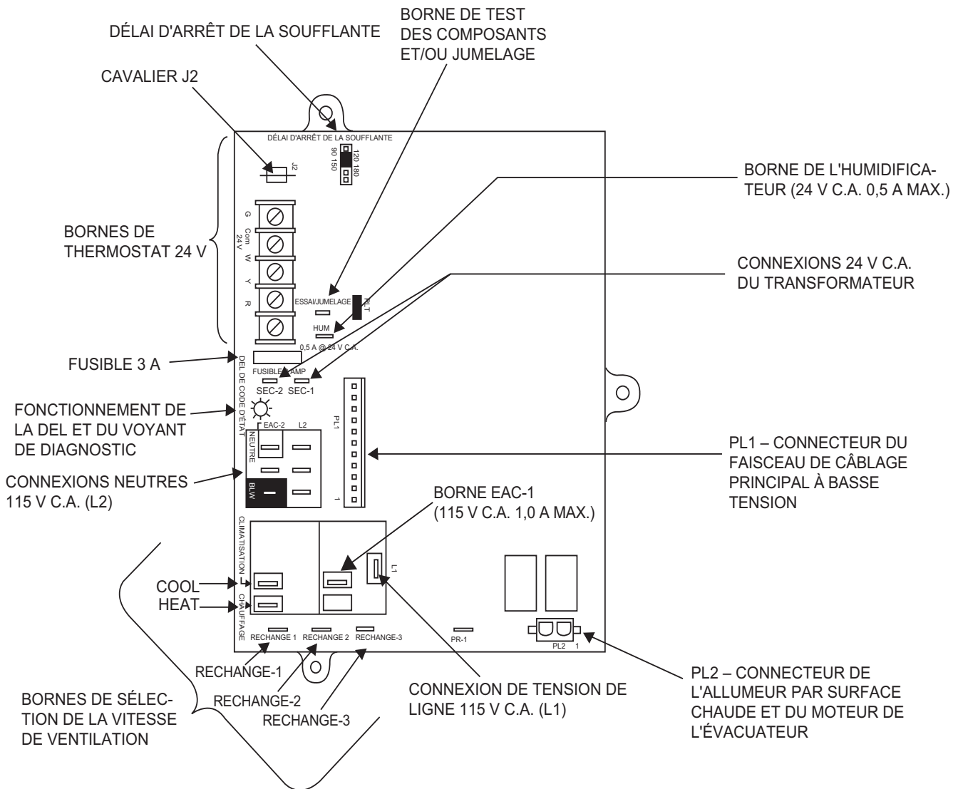
Figure 40 – Exemple de panneau de commande de chaudière à une phase
