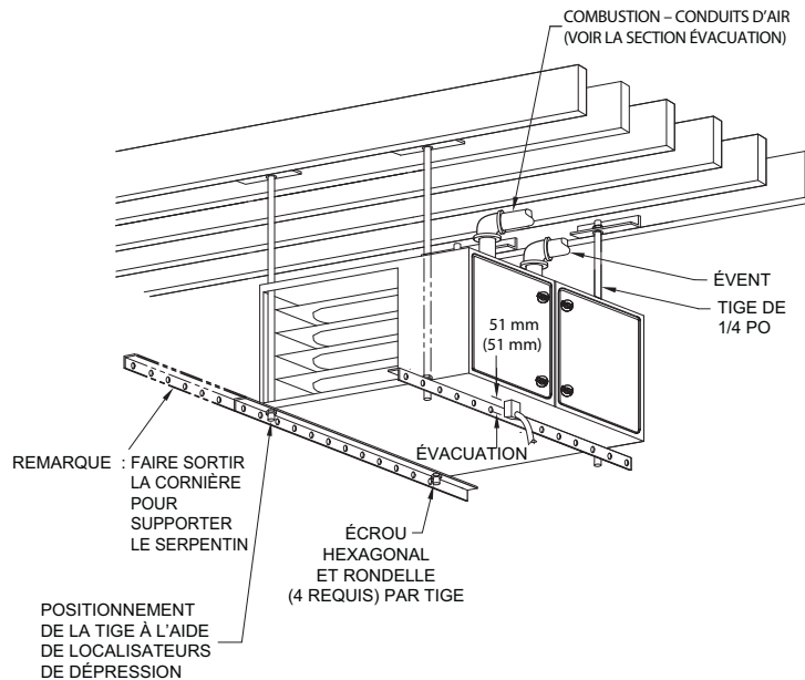
Figure 31 – Plateforme de travail pour installation dans le grenier
