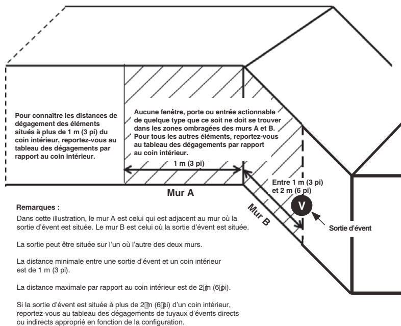
Figure 45 – Sorties dans les coins intérieurs
