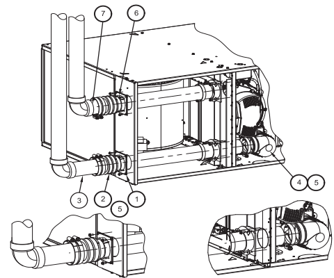
CONFIGURATION HORIZONTALE À DROITE ET VENTILATION VERTICALE
