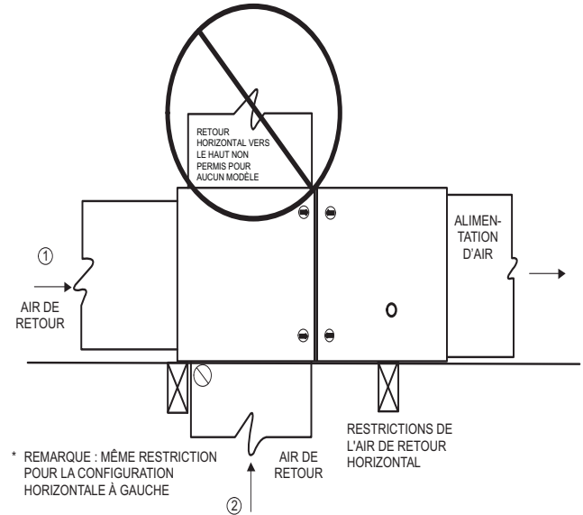
Figure 29 – Configurations et restrictions des conduits de retour d'air horizontaux à droite
