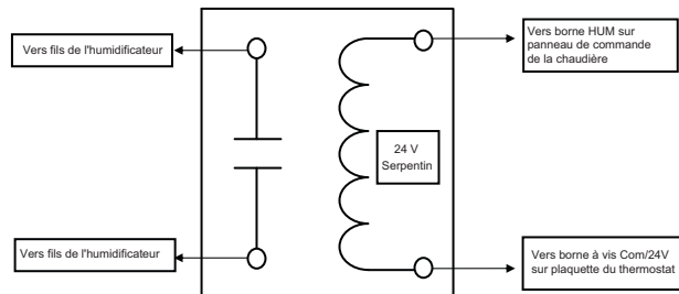
Figure 38 – Relais d'isolation pour humidificateurs, fourni sur place, avec bloc d'alimentation interne
