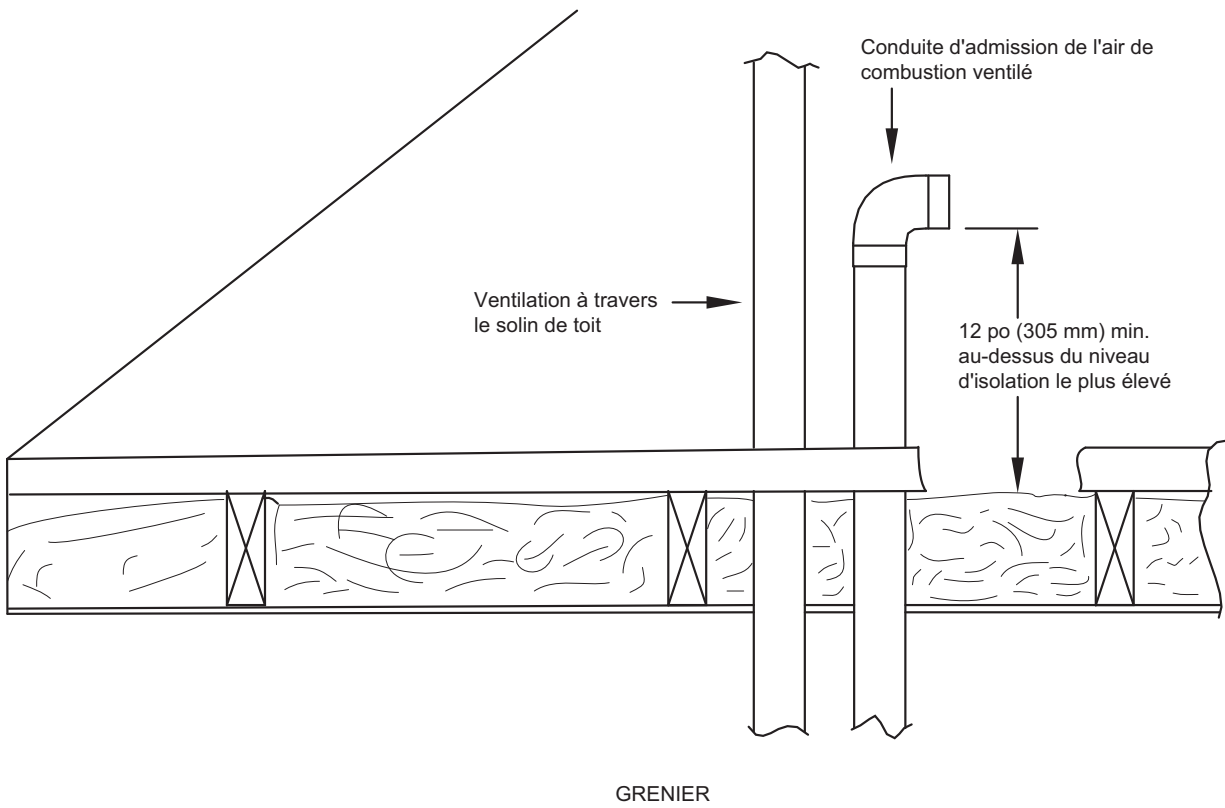
Figure 57 – Sorties d'évent pour système à air de combustion ventilé
