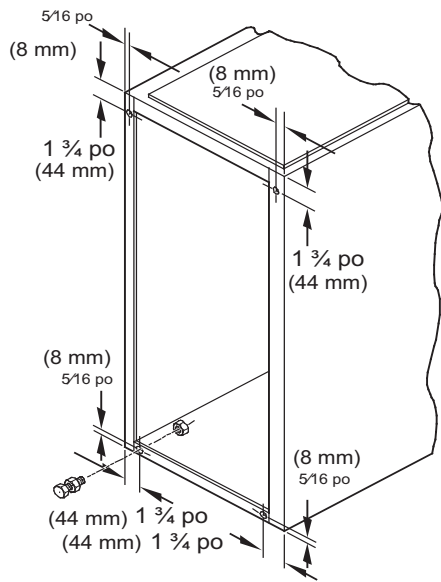
Figure 25 – Pattes de mise à niveau
