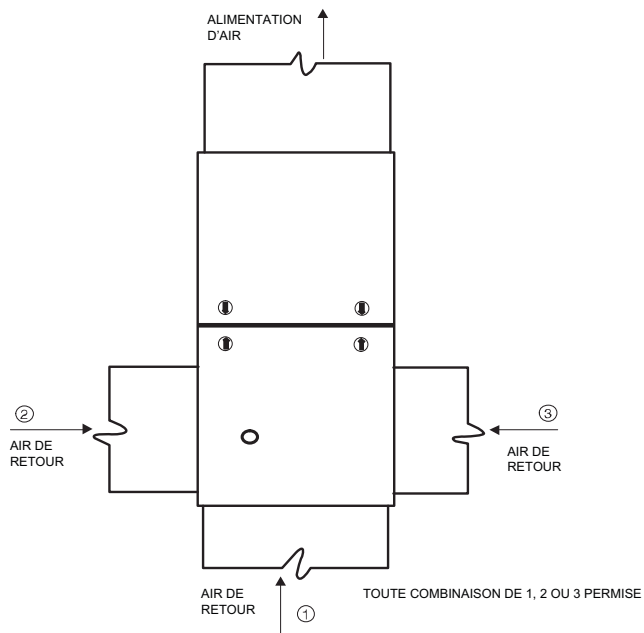
Figure 27 – Configurations et restrictions des conduits de reprise ascendant
