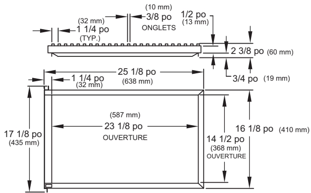
Figure 19 – Support de filtre latéral
