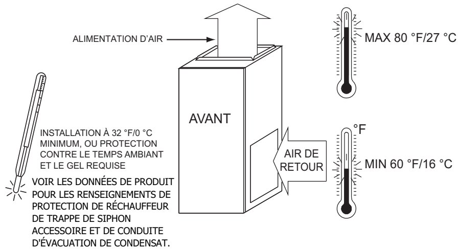
Figure 3 – Protection contre le gel et température de l'air repris
