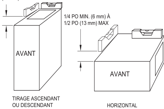
Figure 26 – Exigences d'inclinaison de la chaudière
