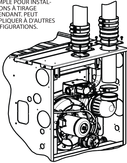
Figure 58 – Exemple de raccordement de tuyau d'entrée d'air pour des systèmes de ventilation en polypropylène
