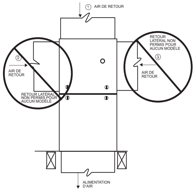
Figure 28 – Configurations et restrictions des conduits de reprise descendant
