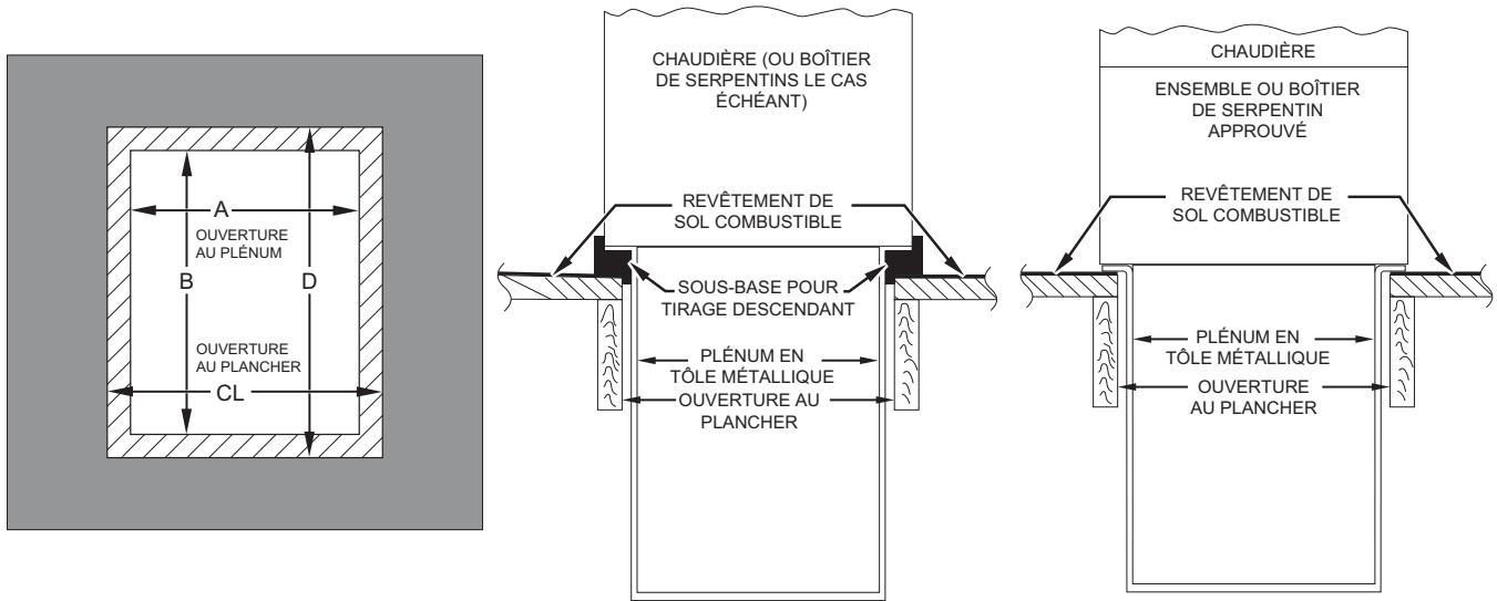
Figure 21 – Installation sur revêtement de plancher combustible
