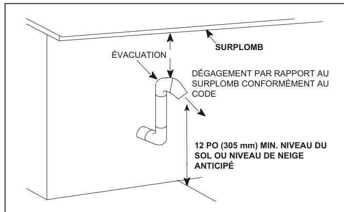
Figure 56 – Sortie d'évent pour l'Alberta et la Saskatchewan
