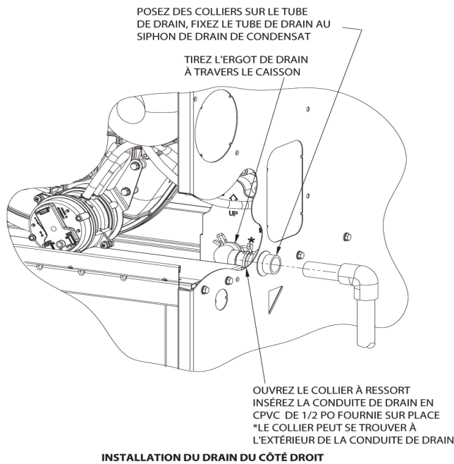
Figure 15 – Œillet d'évacuation de condensat formé en caoutchouc
