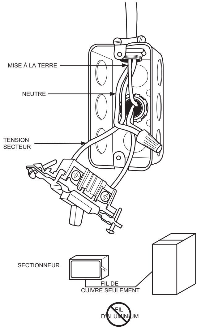
Figure 37 – Coffret électrique externe fourni sur place sur le caisson de la chaudière
