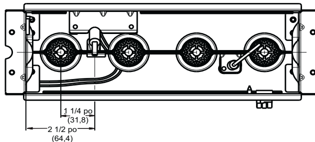
Figure 65 – Position de l'allumeur— vue de dessus
