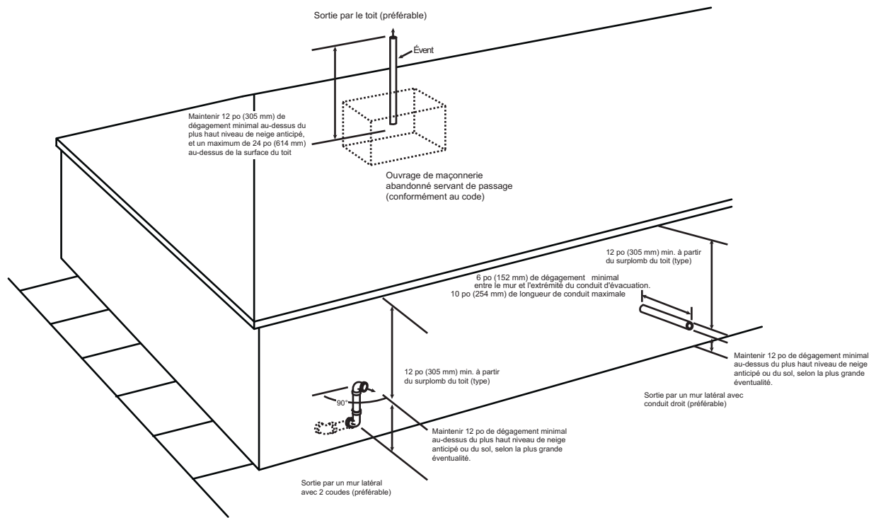
Figure 55 – Sortie d'évent pour système à ventilation non directe et à air de combustion ventilé
