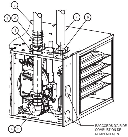
CONFIGURATION HORIZONTALE À DROITE ET VENTILATION VERTICALE
