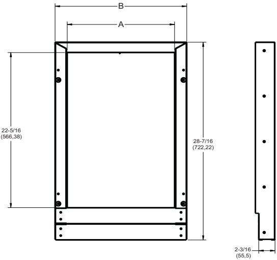
Figure 20 – Filtre du fond
