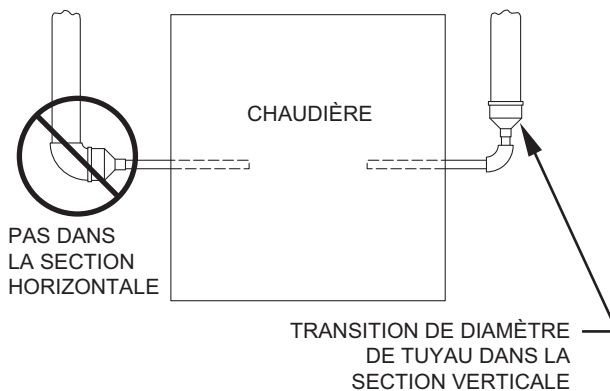
Figure 44 – Emplacement des transitions de diamètre de tuyau de ventilation de l'air de combustion et configuration des coudes
