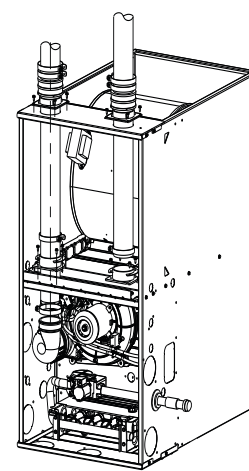
CONFIGURATION VERTICALE À TIRAGE DESCENDANT
