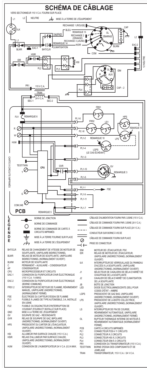
Figure 73 – Schéma de câblage
