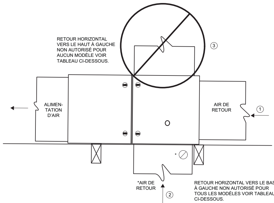
Figure 30 – Configurations et restrictions des conduits de retour d'air horizontaux à gauche
