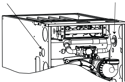
Figure 33 – Entrée de gaz
