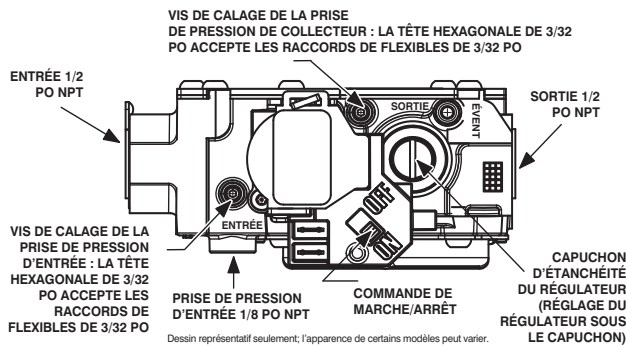
Figure 61 – Vanne de gaz avec orifices de pression
