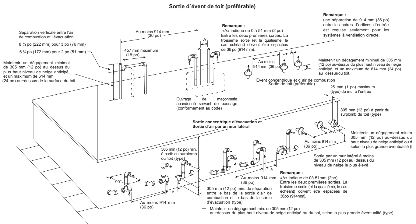
Figure 54 – Air de combustion et sortie d'événement pour système d'évacuation directe (2 tuyaux)
