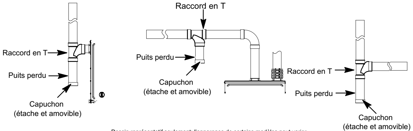
Figure 59 – Siphon à humidité de tuyau d'entrée d'air de combustion recommandé
