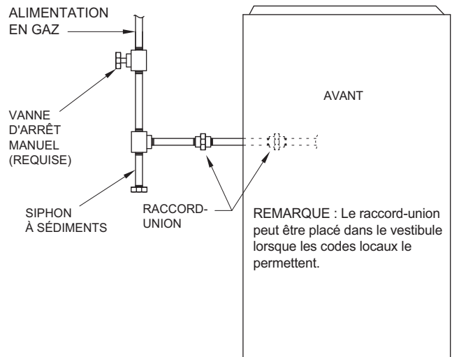
Figure 35 – Disposition type de la tuyauterie de gaz
