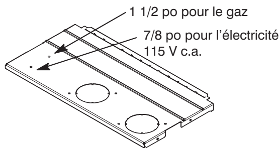
Figure 33 – Entrée de gaz
