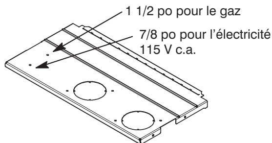
Figure 31 – Entrée de gaz
