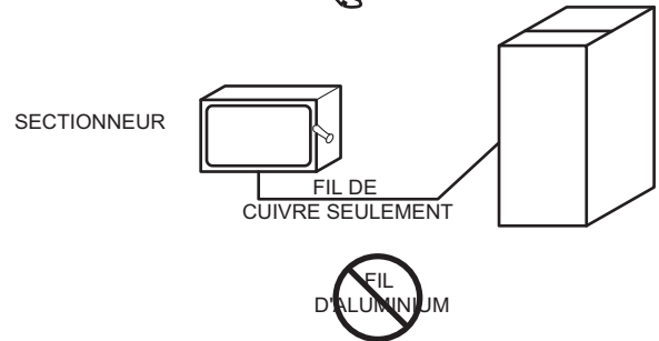
Figure 35 – Coffret électrique externe fourni sur place sur le caisson de la chaudière
