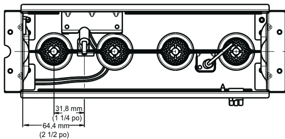
Figure 64 – Position de l'allumeur— vue de dessus
