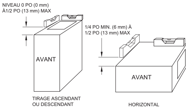
Figure 25 – Exigences d'inclinaison de la chaudière
