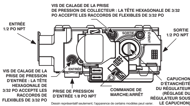
Figure 60 – Vanne de gaz avec orifices de pression
