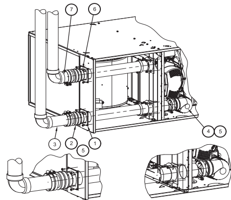
CONFIGURATION HORIZONTALE À DROITE ET VENTILATION VERTICALE
