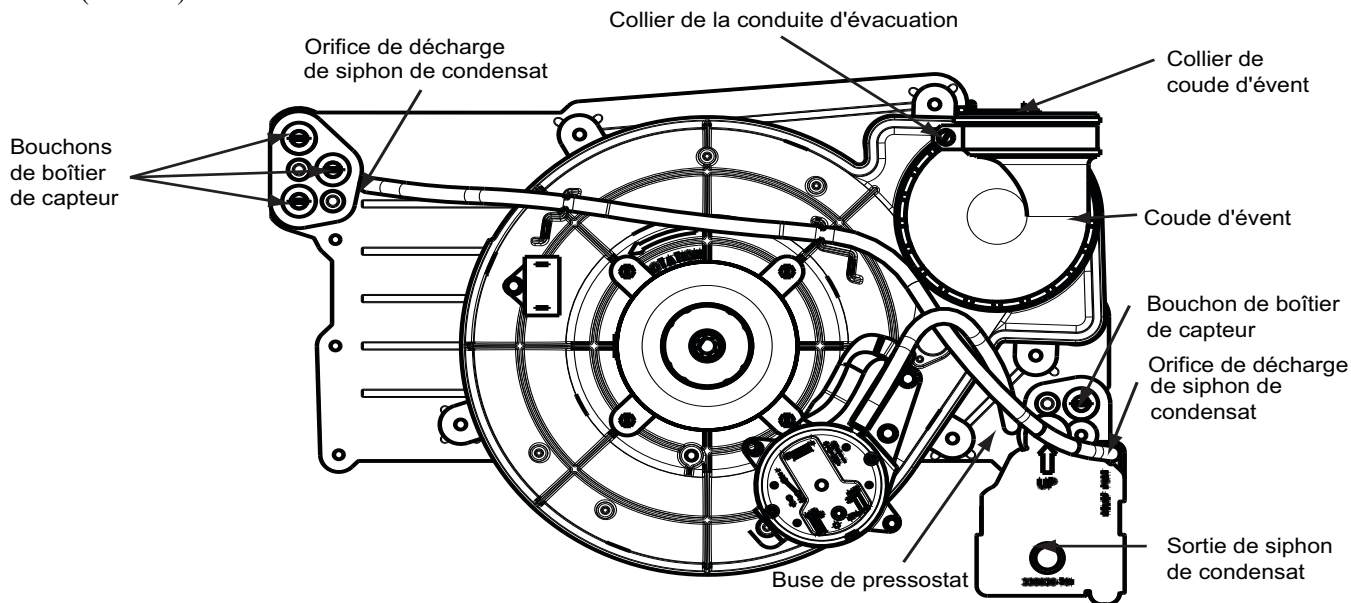
CONFIGURATION DE SIPHON À TIRAGE ASCENDANT
