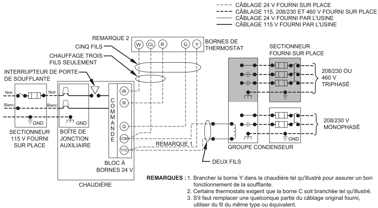
Figure 37 – Schéma de câblage type d'un appareil à une phase
