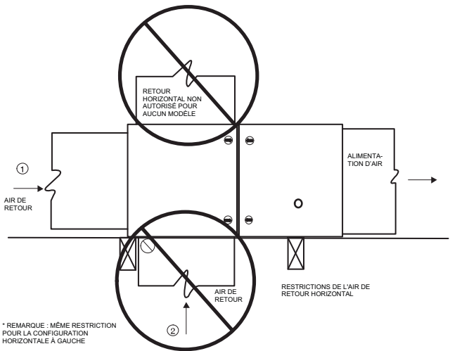
Figure 28 – Configurations et restrictions des conduits de reprise horizontaux
