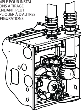
Figure 57 – Exemple de raccordement de tuyau d'entrée d'air pour des systèmes de ventilation en polypropylène
