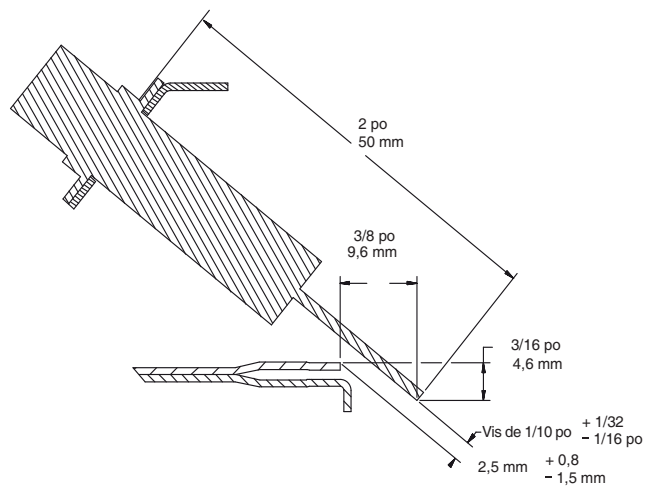
Figure 65 – Position de l'allumeur— vue de côté
