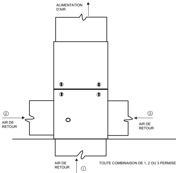
Figure 26 – Configurations et restrictions des conduits de reprise ascendant
