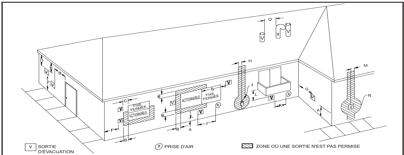
Figure 50 – Fixation du tuyau d'air de combustion
