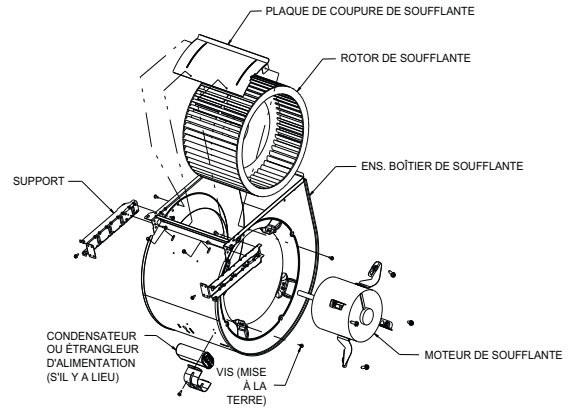
Figure 69 – Ensemble de soufflante
