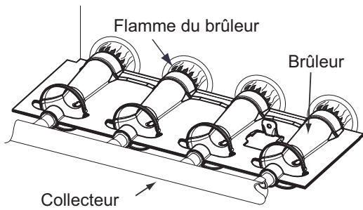
Figure 68 – Flamme du brûleur
