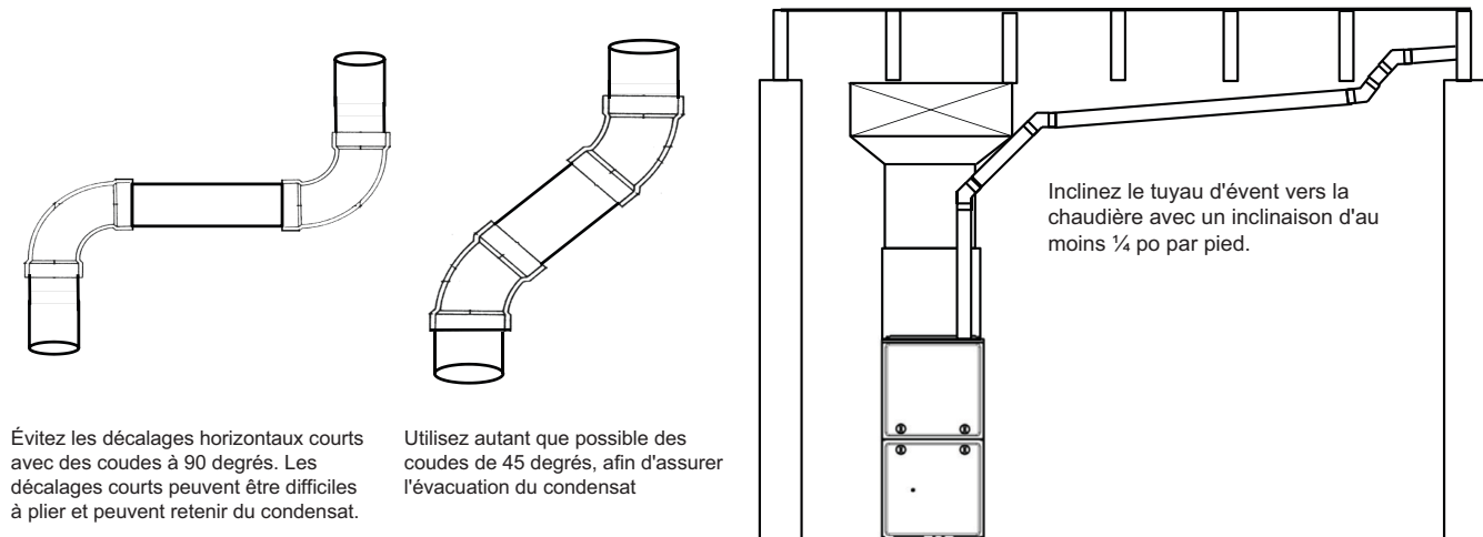
Figure 42 – Raccordement des événements près de la chaudière
