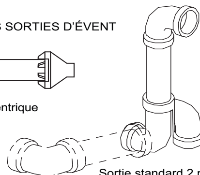
Sortie standard 2 po, 3 po, ou optionnelle 4 po
