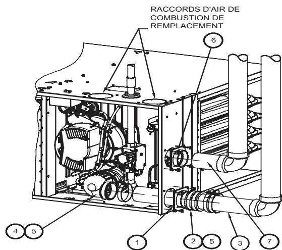
CONFIGURATION HORIZONTALE À DROITE ET VENTILATION À DROITE
