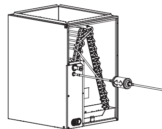
Fig. 7 – Déshydrateur-filtre de la conduite de liquide
