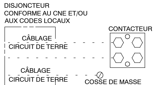
Fig. 9 – Raccords de conduite
