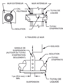
Fig. 1 – Installation des conduites
