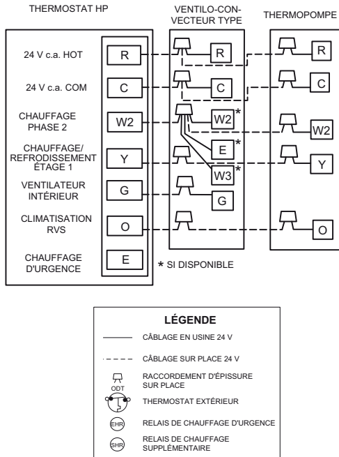
Fig. 10 – Schémas de câblage génériques (consultez les instructions d'installation du thermostat pour connaître les combinaisons spécifiques des appareils)
