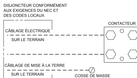
Fig. 8 – Raccords de conduite
