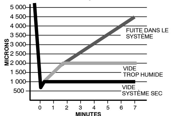
Fig. 7 – Courbe de vide
