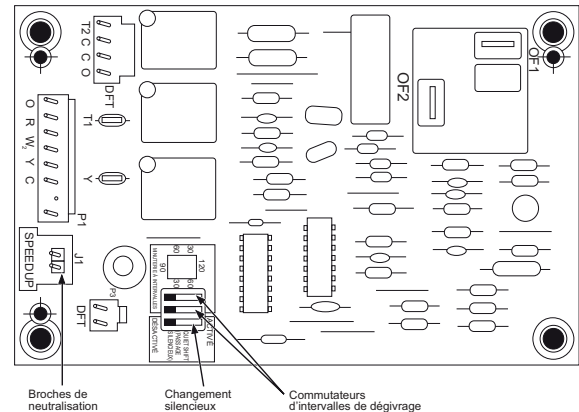
Fig. 11 – Commande de dégivrage
