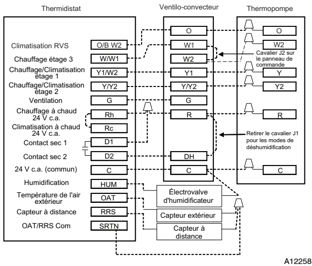
Fig. 9 – Câblage du thermostat avec ventil-convecteur et thermopompe à 2 étages
