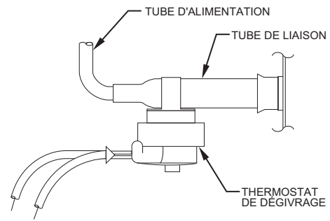
Fig. 3 – Emplacement du thermostat de dégivrage
