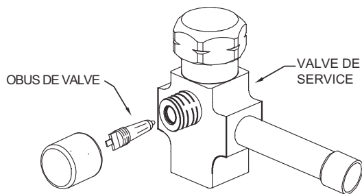
Fig. 5 – Valve de service de vapeur
