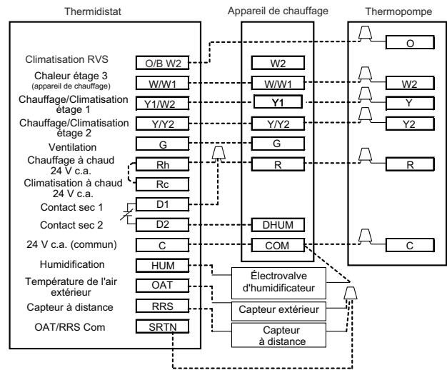
Fig. 10 – Thermostat avec appareil de chauffage à vitesse variable et thermopompe à 2 étages
