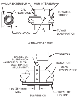
Fig. 1 – Installation de la tuyauterie
