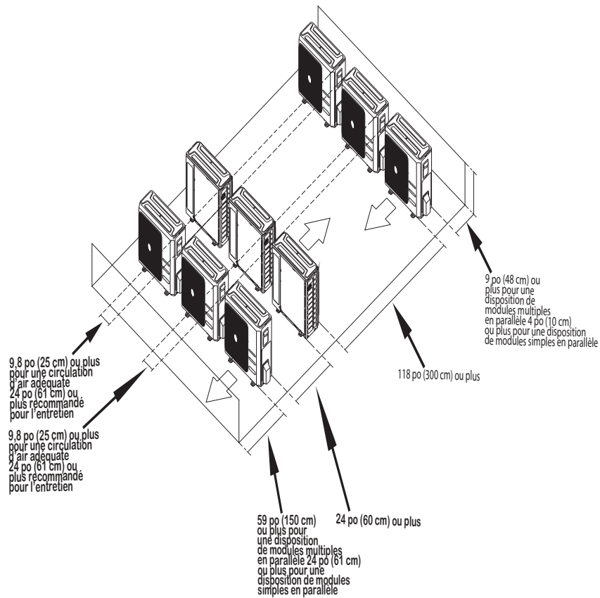
Figure 6 – Dégagements des modules multiples
