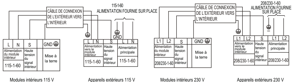
Figure 14 – Schémas de connexion
