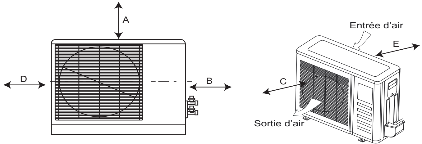
Figure 5 – Dégagement de l'appareil extérieur
