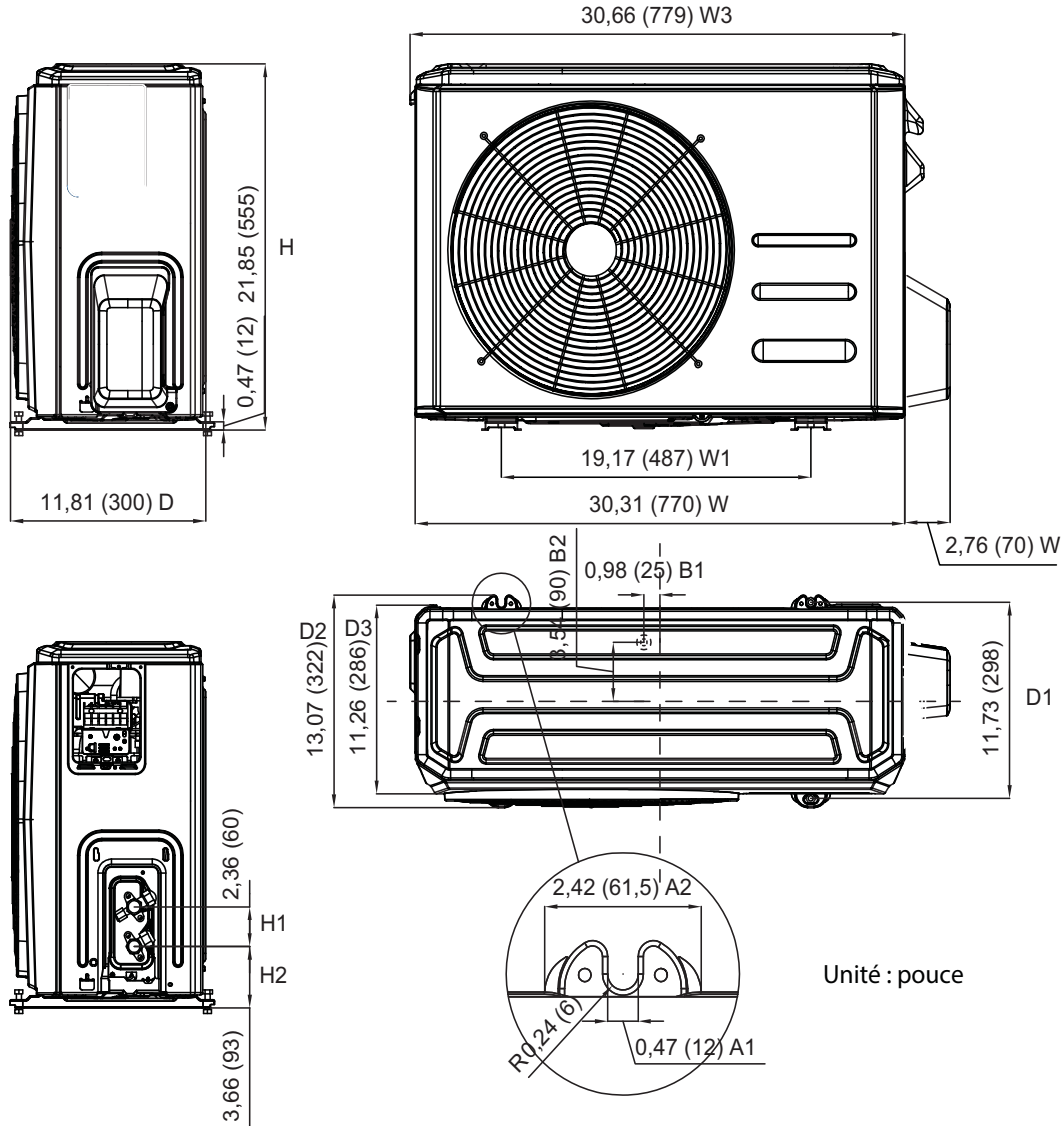
Figure 2 – Capacités 9 000 et 12 000 Thermopompe et Capacité 18K Refroidissement seulement
