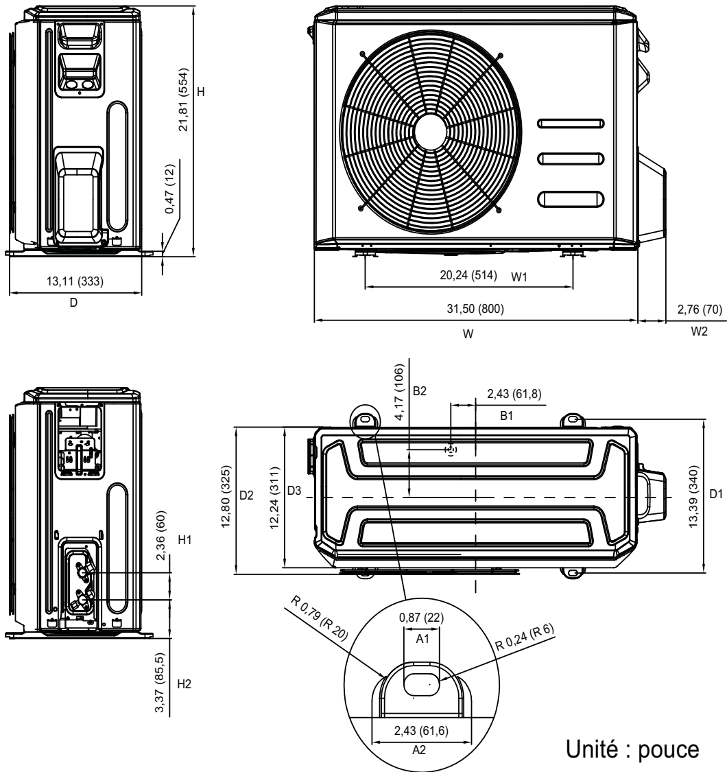
Figure 3 – Capacité 18K thermopompe
