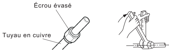
Figure 11 – Serrez l'écrou évasé.
