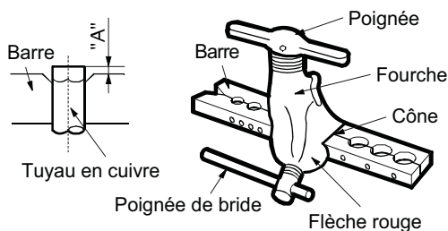
Figure 16 – Outil à évaser
