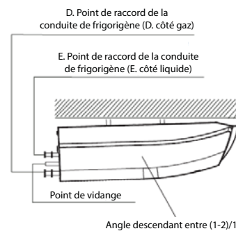
Figure 13 – Installation au plafond
