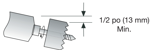
Figure 18 – Perçage des trous
