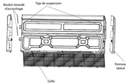
Figure 10 – Retrait des panneaux latéraux et de la grille
