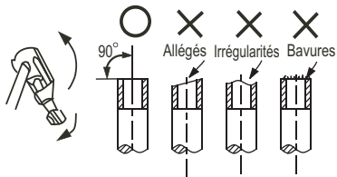
Figure 15 – Coupe du tuyau
