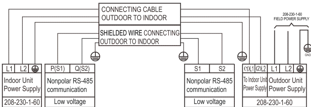
Figure 24 – Schémas de raccordement – capacités 36 et 58
