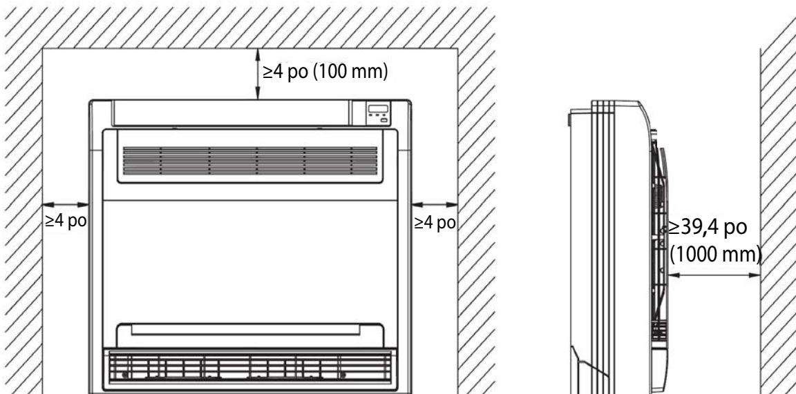
Figure 4 – Dégage ment du module intérieur
