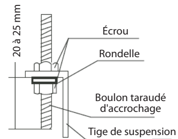
Figure 11 – Repérage de la tige de suspension
