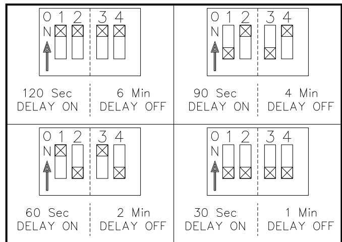
Figure 9 : Délais de départ et d'arrêt du ventilateur Carte#1158
