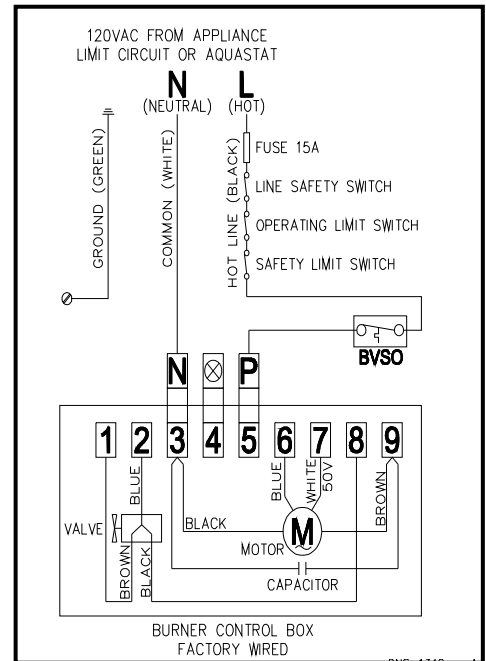
Riello Burner
