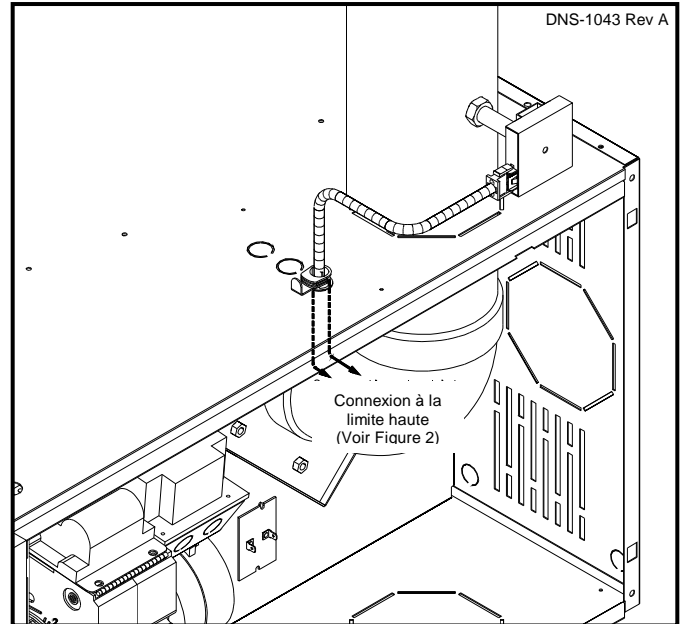
Figure 7 : Branchement dispositif anti-refoulement, installation horizontale avec évacuation verticale
