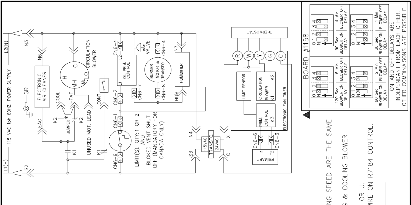
Figure 12 : Diagramme électrique, brûleur Beckett
