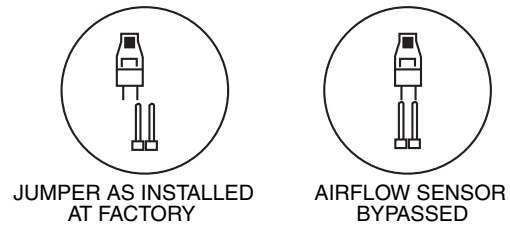
Fig. 4 - JP9 Prongs
