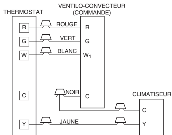
Fig. 6 - Agencement du câblage – Climatiseur (refroidissement et chauffage 1 étage)
