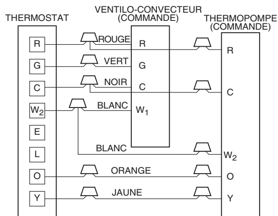
Fig. 7 - Agencement du câblage – Thermopompe (refroidissement et chauffage 2 étages)
