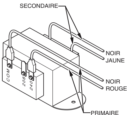
Fig. 5 - Connexions du transformateur
