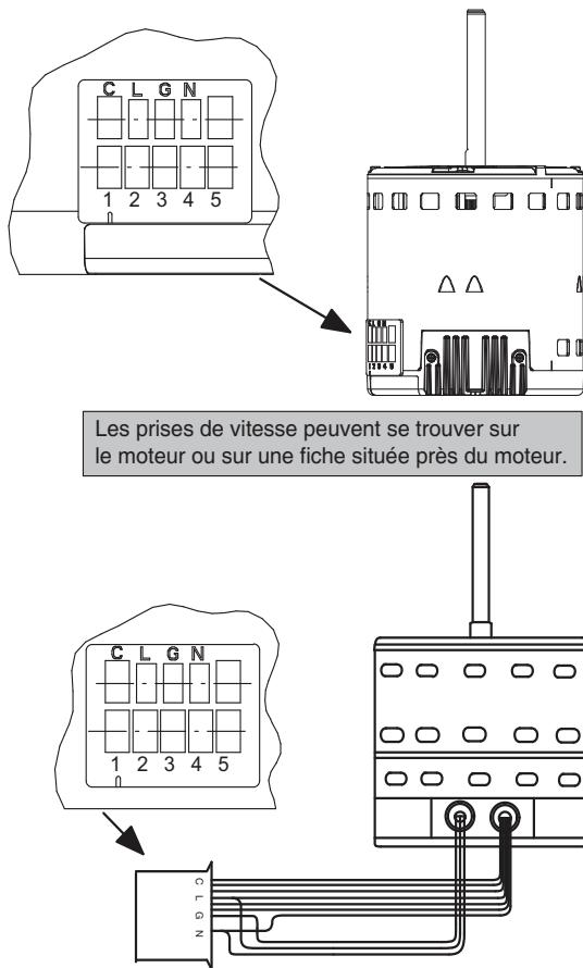
Fig. 8 - Prises de vitesse des moteurs ECM (tailles 19, 25, 31 et 37)
