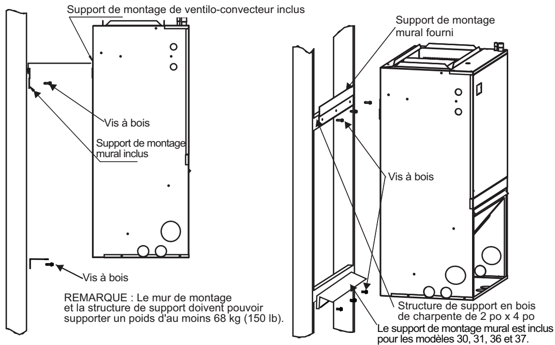
Fig. 3 - Installation pour montage mural
