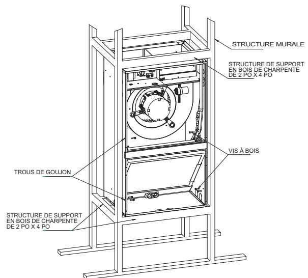
Fig. 4 - Montage dans un bâti
