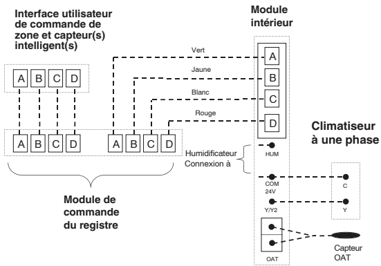
Schéma de connexion de zonage pour l'appareil de chauffage ou le ventilo-convecteur FE avec climatiseur à 1 phase non communicant
