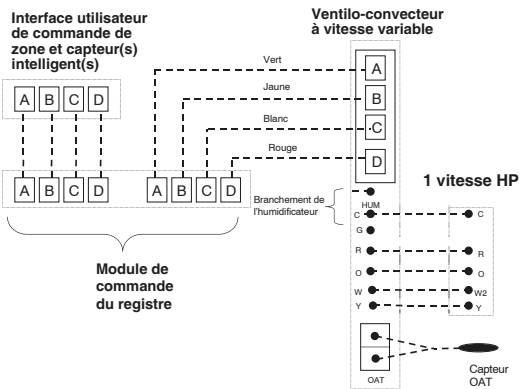
Schéma de connexion de zonage pour le ventilo-convecteur FE avec thermopompe à 1 phase non communicante
