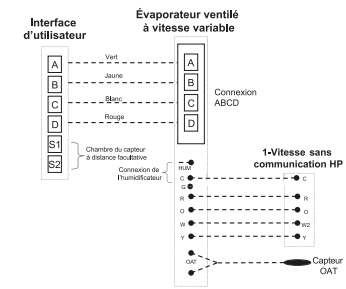
Fig. 4 - Diagramme de connexion pour fournaise ou évaporateur ventilé FE sans communication 1 - Stage HP
