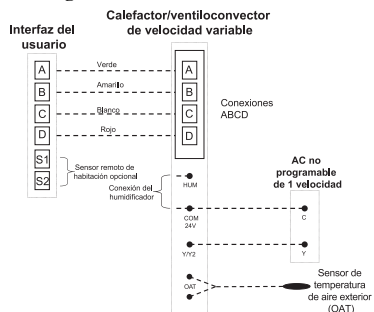
Fig. 2 - Diagrama de la conexión de cuatroalambres
