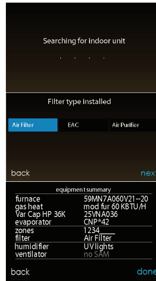
Fig. 5 - Secuencia de encendido
