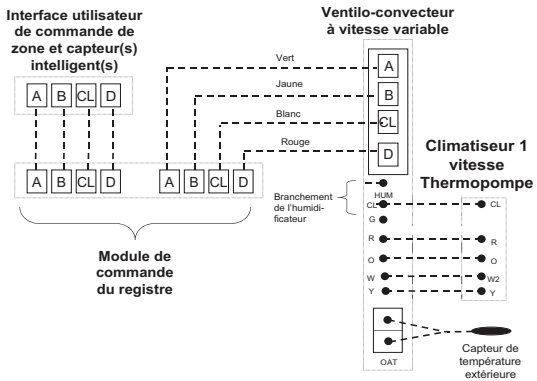
Schéma de connexion de zonage pour le ventilo-convecteur FE avec thermopompe à 1 phase non communicante
