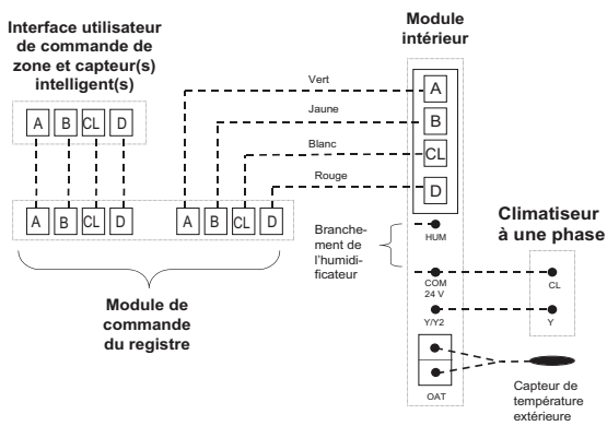
Schéma de connexion de zonage pour la fournaise ou le ventilo-convecteur FE avec climatiseur à 1 phase non communicant
