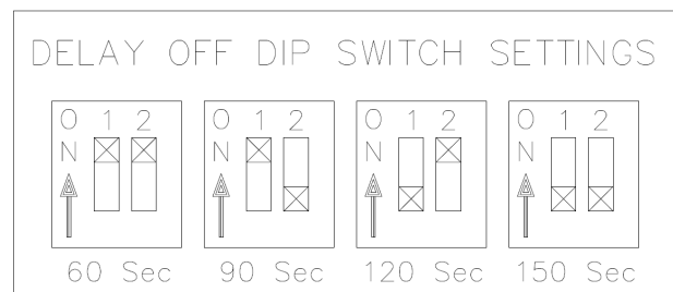
Figure 8 – Délais d'arrêt du ventilateur-Carte #9103A
