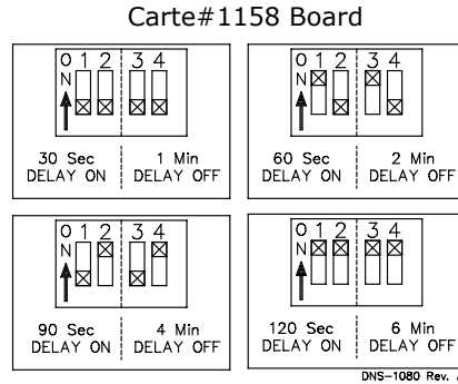
Figure 9 – Délais de départ et d'arrêt du ventilateur-Carte #1158
