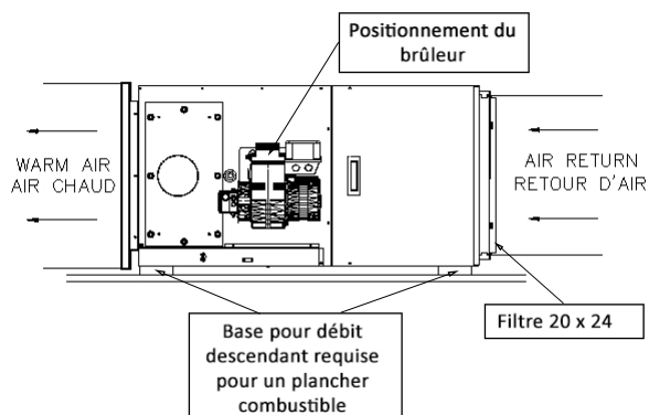
Figure 4 – Débit horizontal
