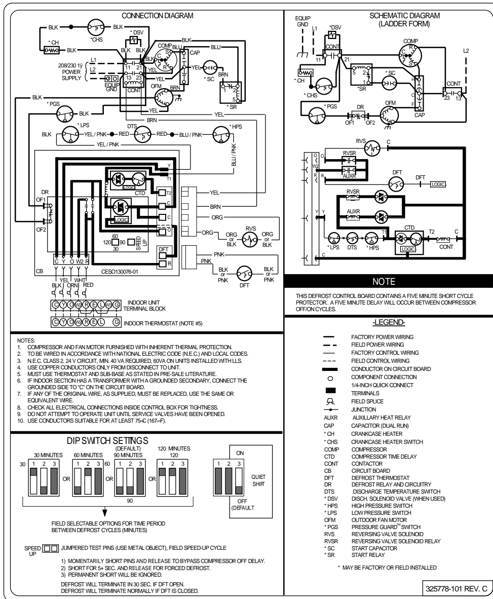
Fig. 2—38SYG060; 208-230v; 1 Phase; 60 Hertz
