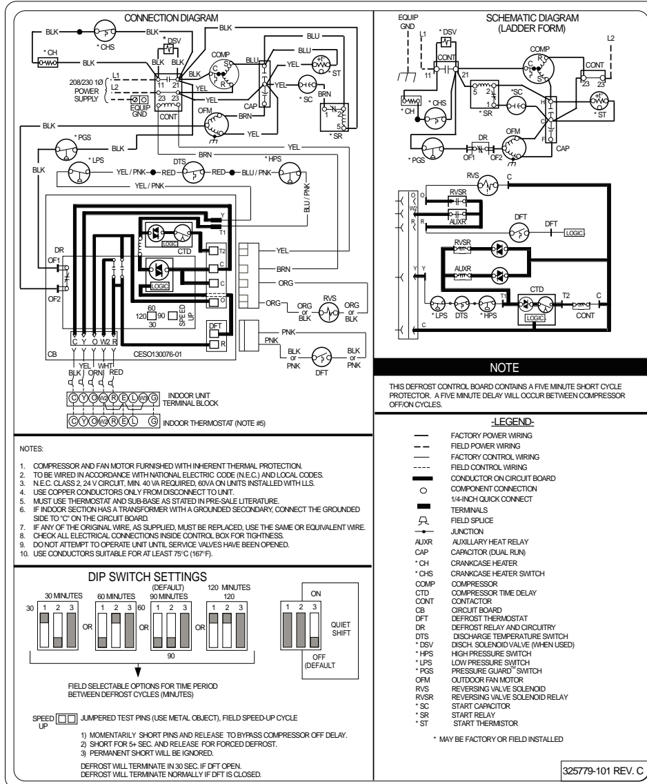
Fig. 1—38SYG018-048; 208-230v; 1 Phase; 60 Hertz
